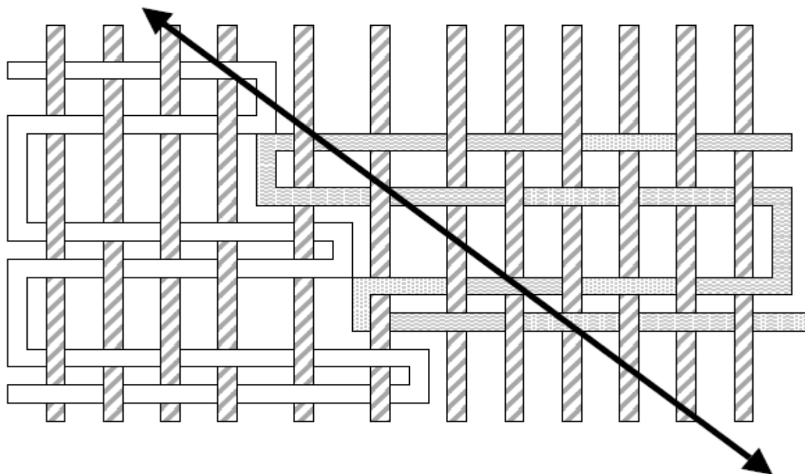
الگوی بافت متصل مورب با تار مشترک
