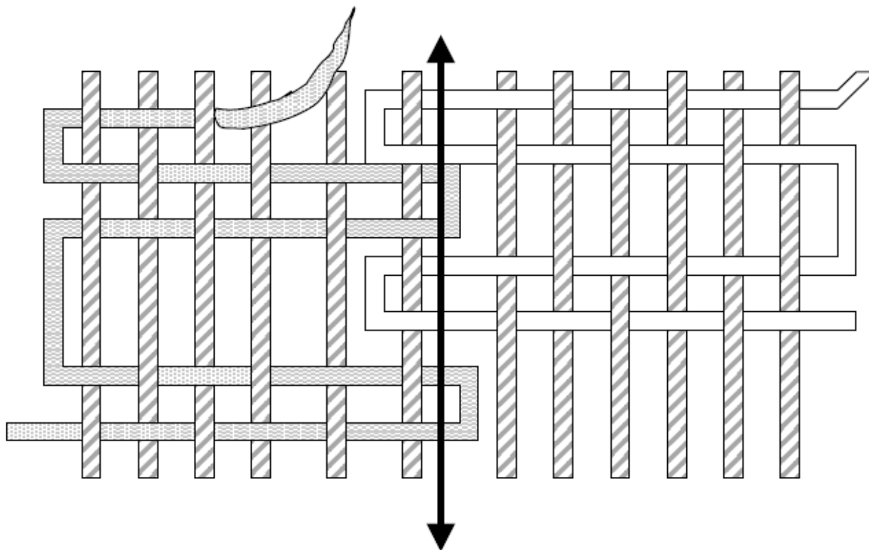
الگوی بافت متصل مورب با تار مشترک
