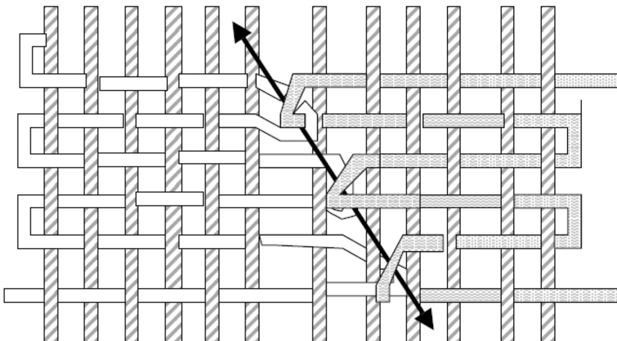
الگوی بافت متصل مورب با پود مشترک
